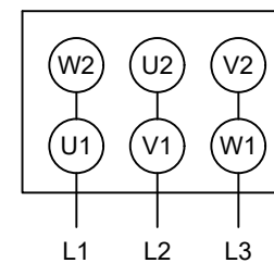
CABLAGE DU MOTEUR EN TRIANGE
